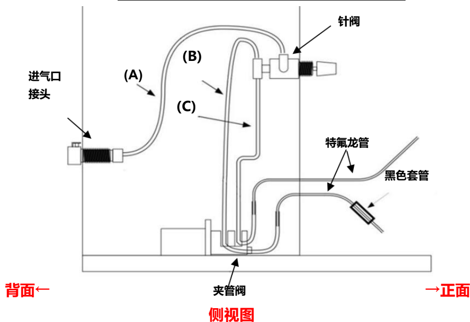
RRDE-3A 内部管路图 (侧视图)
